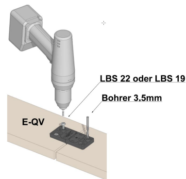
E-QV Querverbinder 2-teilig
